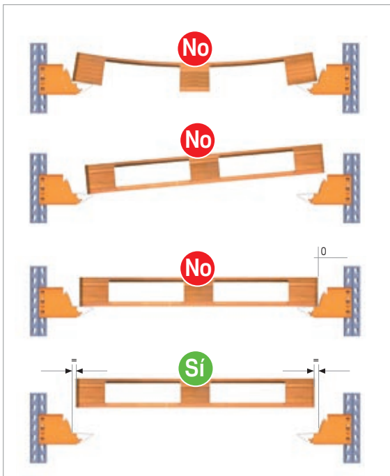
Posicionar los pallets en la dirección adecuada.
