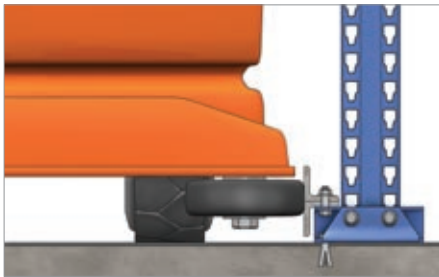
Carril guía.
