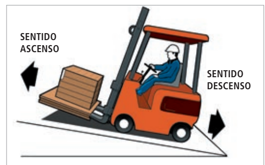
Figura 3 Circulación en pendientes.
