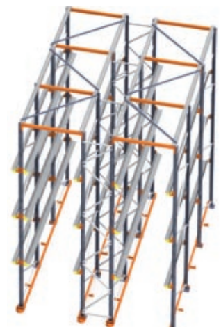
Atirantados.
