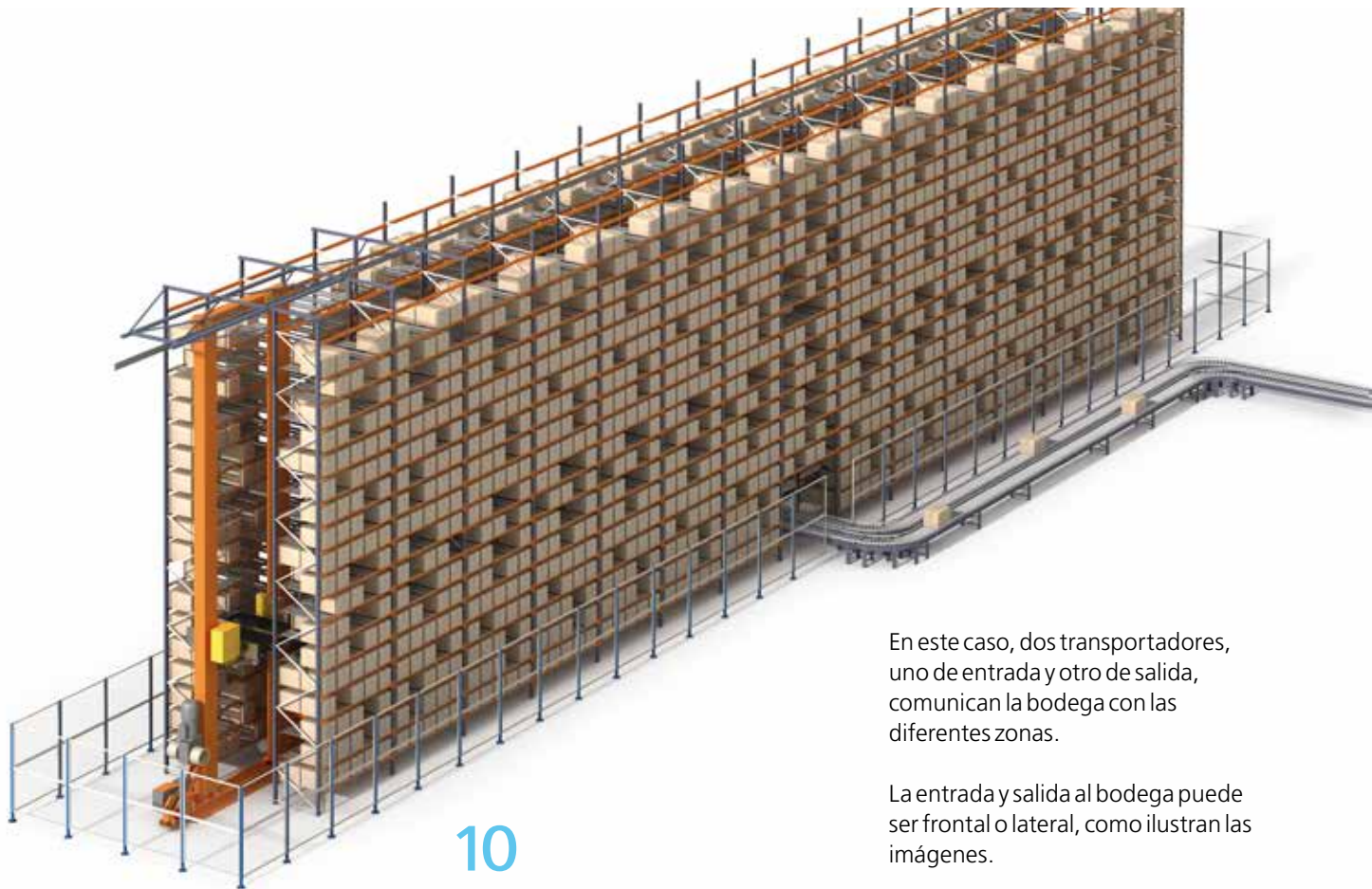
Bodega automática para cajas de cartón con entrada y salida lateral.
