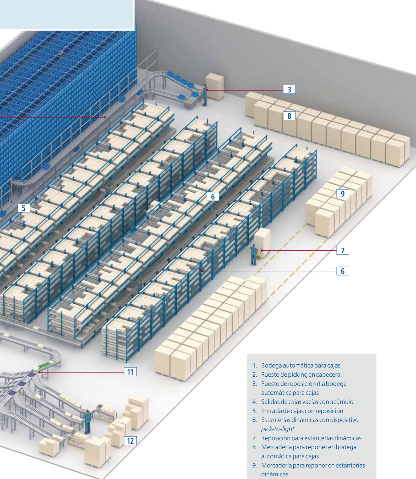
Bodega automática para cajas combinado con estanterías dinámicas y un clasificador de pedidos.
